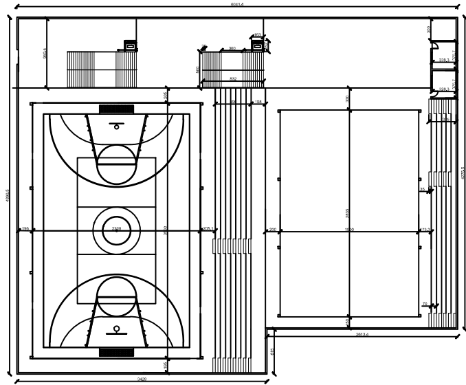
PLANTA BAIXA
