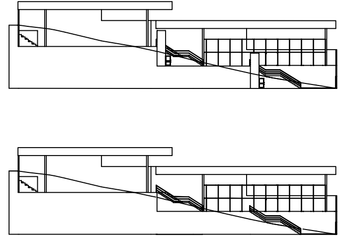
CORTE TRANSVERSAL
